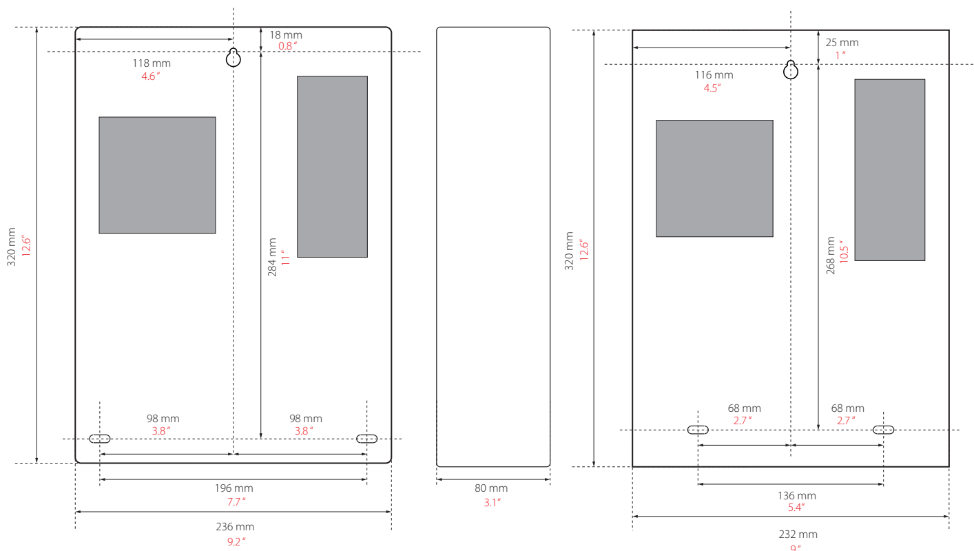
2A/12V DC strömförsörjning - apparatlåda av plast 857-250
